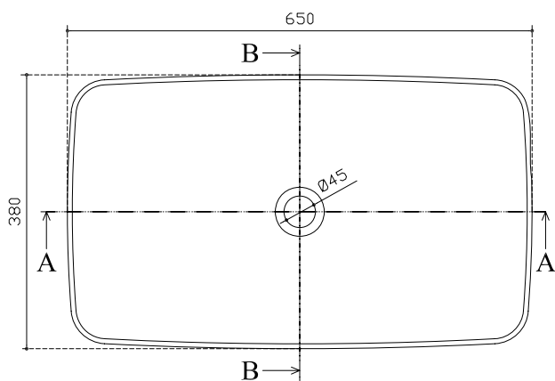
Vista dall'alto View from above Vista desde arriba Vue de dessus
