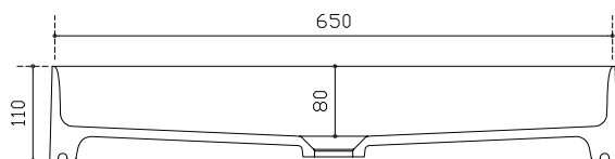
Sezione A-A Section A-A Sección A-A Section A-A
