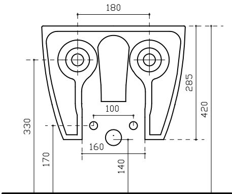
Vista posteriore
